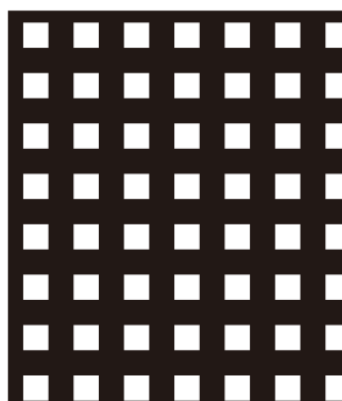
103 3.0□×6.0P 開孔率 25.0%
