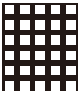
106 5.0□×8.0P 開孔率 39.0%
