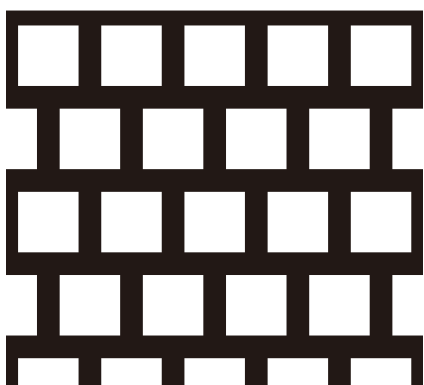
109 8.0□×11.0P 開孔率 52.9%
