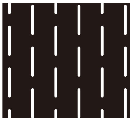
89 (1.2 × 13.0) × (20.0 × 18.0)P 開孔率 8.5%
