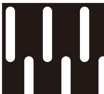
92 (5.0 × 30.0) × (20.0 × 53.8)P 開孔率 27.7%
